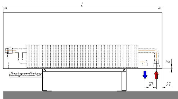
Монтажная схема напольного конвектора "Элегант - плюс 80x250-1то нв (рв)" с нижним подключением (присоединительная резьба - 1/2" внутр.)
