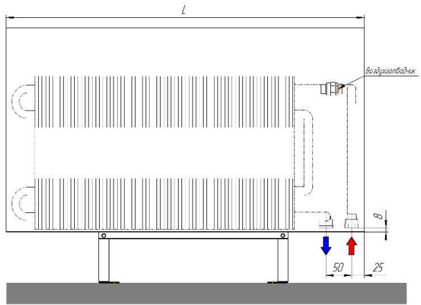
Монтажная схема напольного конвектора "Элегант - Плюс 180xH-6то нв (рв)" с нижним подключением (присоединительная резьба - 1/2" внутр.)
