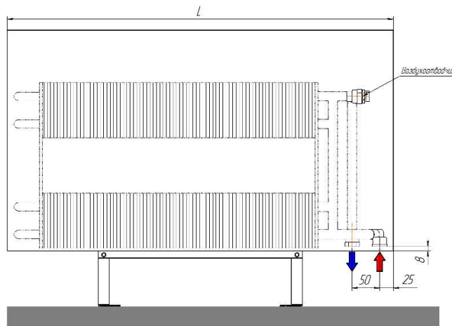
Монтажная схема напольного конвектора "Элегант - плюс 130xH-4то нв (рв)" с нижним подключением (присоединительная резьба - 1/2" внутр.)
