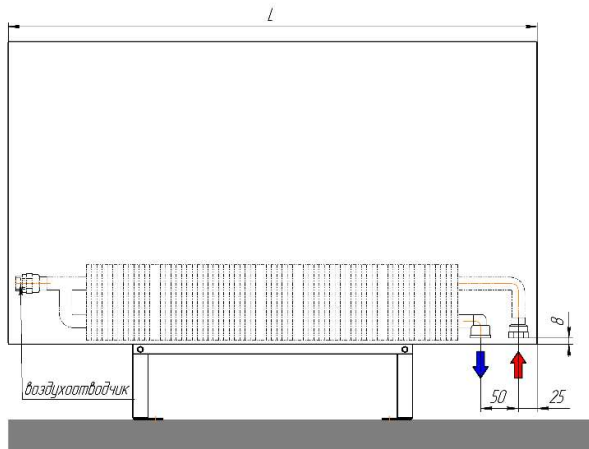
Монтажная схема напольного конвектора "Элегант - плюс 80x400-1то нв (рв)" с нижним подключением (присоединительная резьба - 1/2" внутр.)
