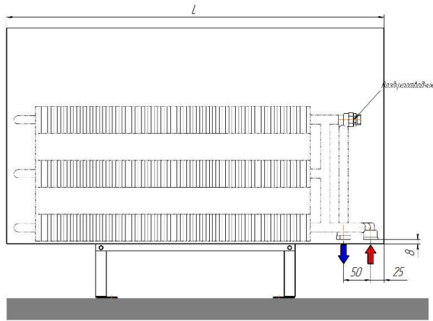
Монтажная схема напольного конвектора "Элегант - плюс 130xH-3то нв (рв)" с нижним подключением (присоединительная резьба - 1/2" внутр.)
