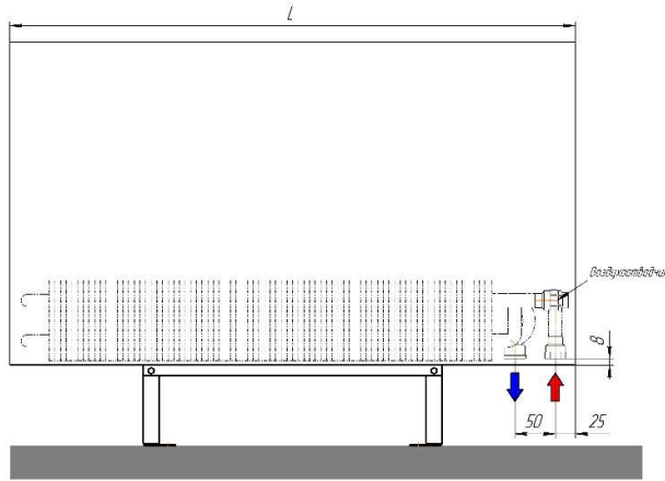
Монтажная схема напольного конвектора "Элегант - Плюс 180xH-3то нв (рв)" с нижним подключением (присоединительная резьба - 1/2" внутр.)
