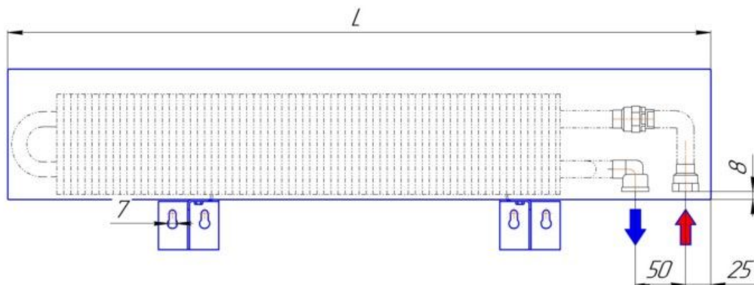
Монтажная схема настенного конвектора "Элегант - мини 230x130-4то Стен" (присоединительная резьба - 1/2")
