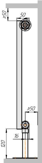
Гармония А 20-1 нп нв
