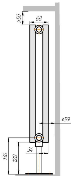
Гармония А 20-2 нв
