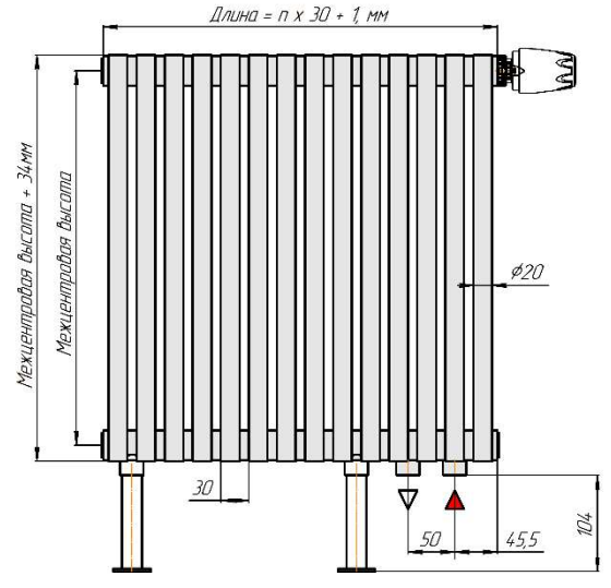
Присоединительная резьба - G 1/2" внутр.
