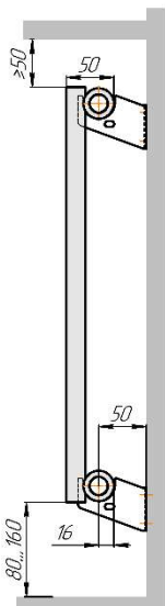
Гармония А 20-1 кронштейн Г-50
