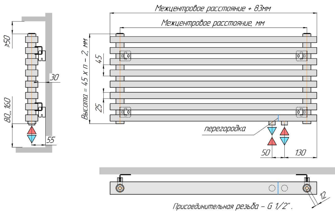
Настенный радиатор QUADRUM NEO 50 H ... R, с правосторонним нижним подключением под арматуру 50 мм (левостороннее нижнее подключение (L) – зеркально)
