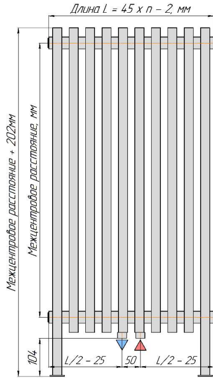
QUADRUN NEO 50 V... CR FF (подача - справа)
