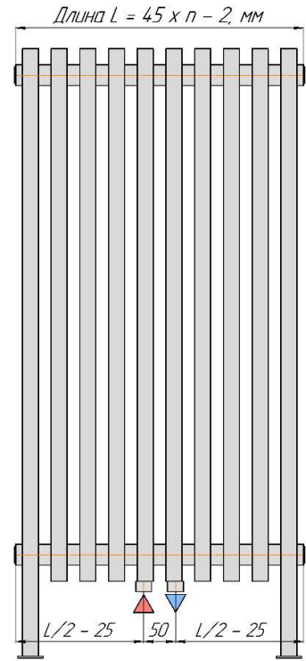
QUADRUN NEO 50 V... CL FF (подача - слева)
