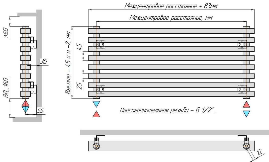
Настенный радиатор QUADRUM NEO 50 H, с разнесенным (седловым) нижним подключением.
