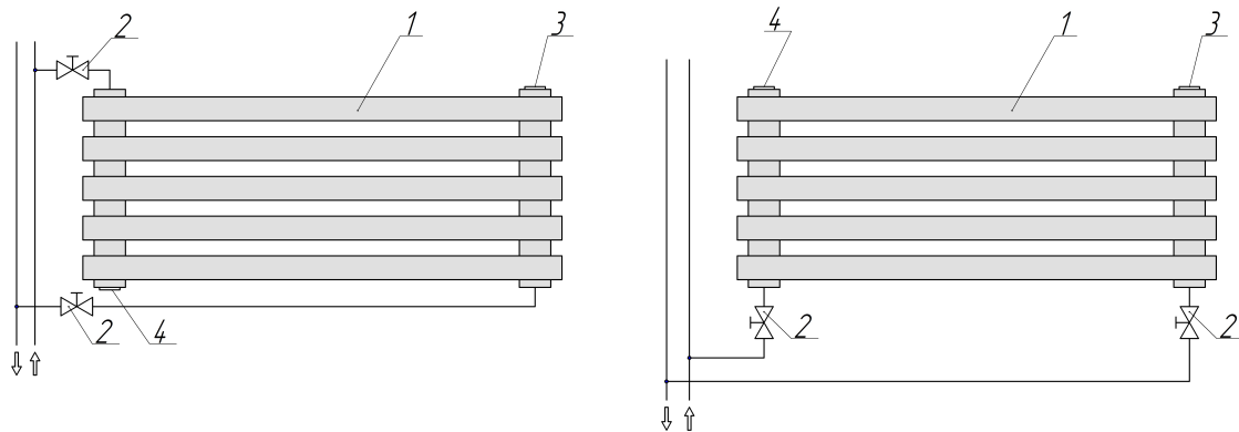
Рис. 3 1. Радиатор. 2. Вентиль (кран). 3. Кран-воздухоотводчик. 4. Пробка глухая.
