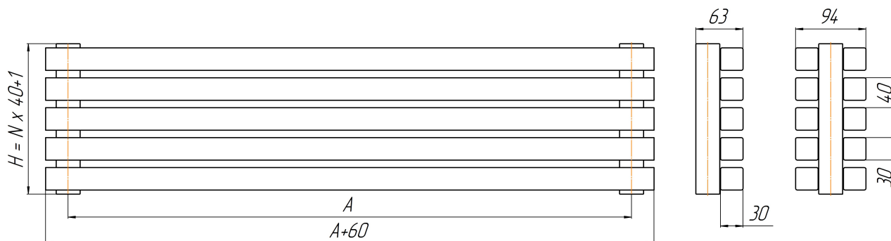
Рис. 1. А – межцентровый (монтажный) размер, N – количество секций.
